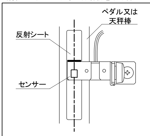
図 3. 4 - 3 反射シートの貼り付け
